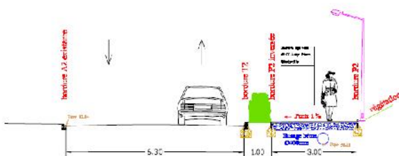
Profil AA
