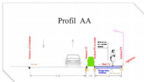
Aménagement de la RD 304 avec piste réservée aux cyclistes et aux piétons
